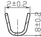
B-B
